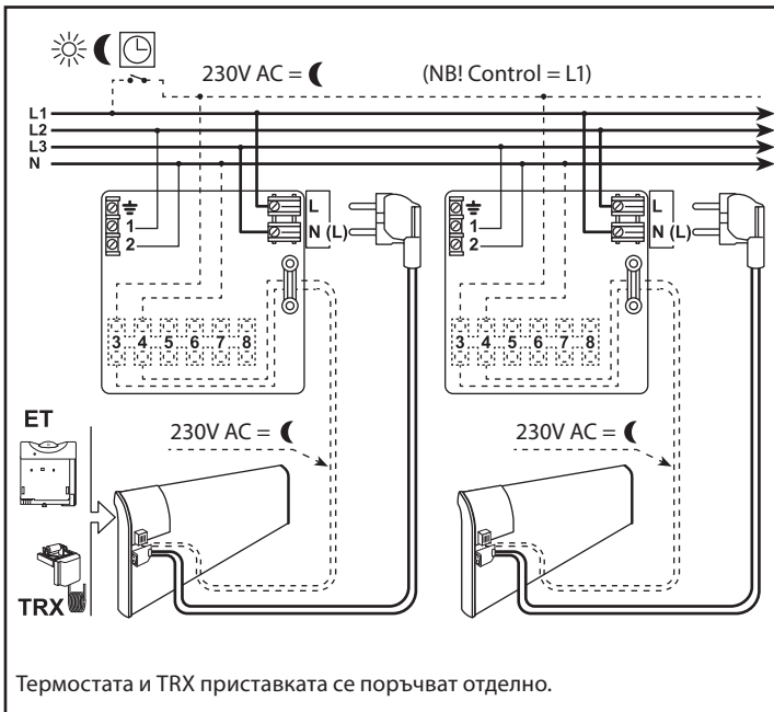
400V схема
