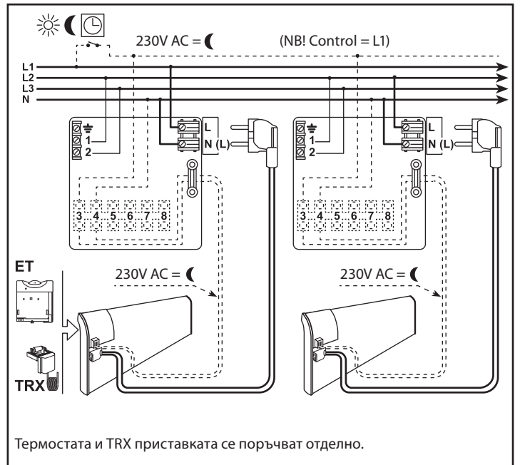
230V схема
